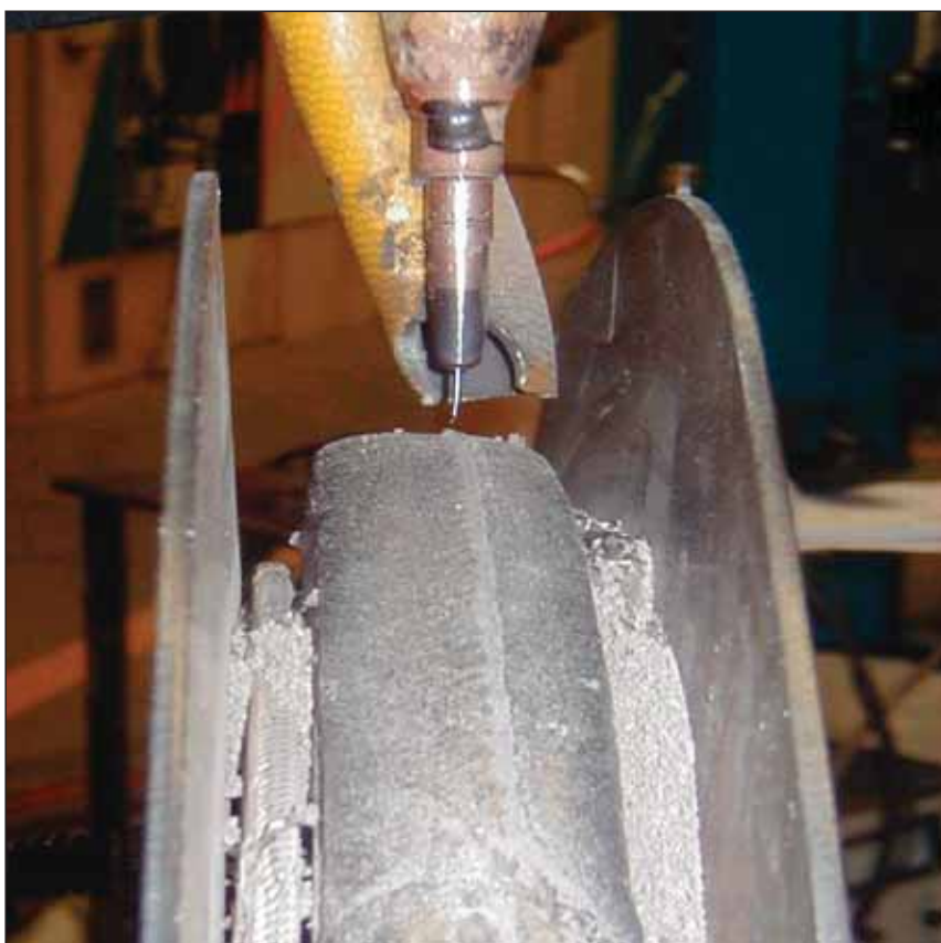
Rechargement fil fourré sous flux.
